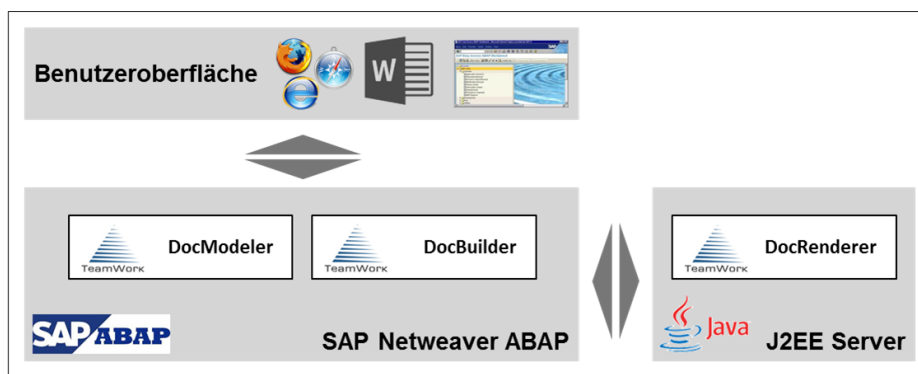
DocBuilder - Architektur
